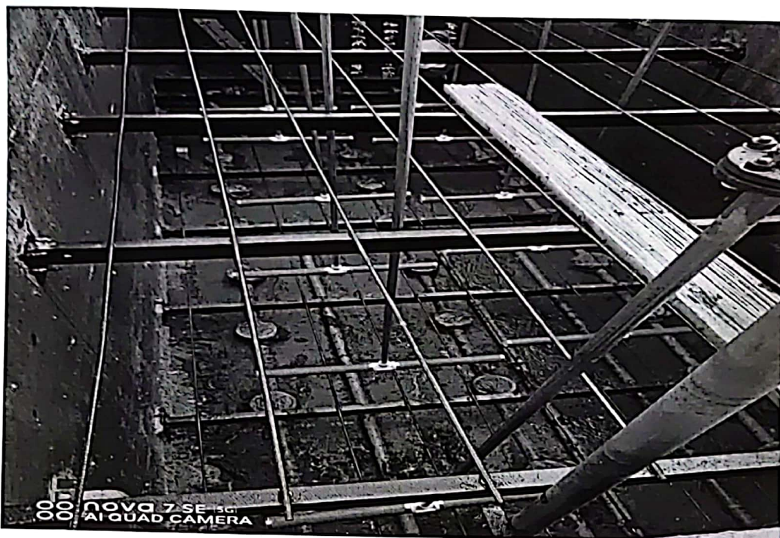
整改后 A/O 池、低负荷池增挂填料、爆气管、盘
