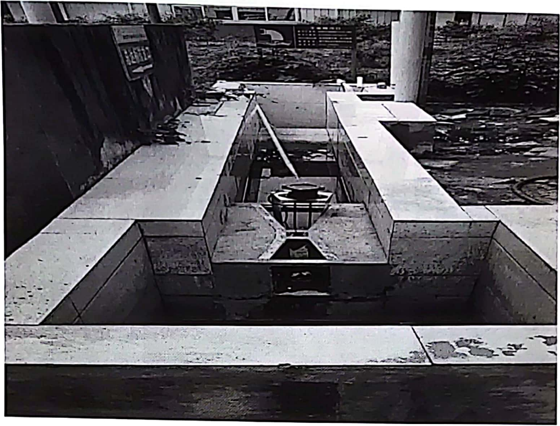
整改后增加巴歇尔槽流量计
